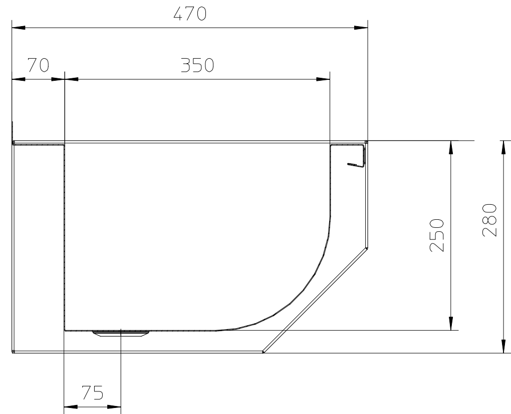
Schnitt D-D
